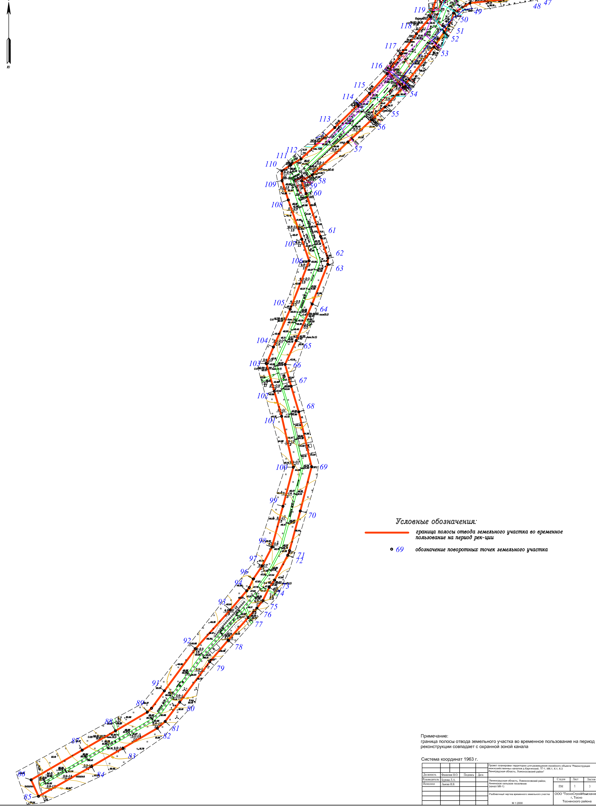
Разбивочный чертеж временного земельного участка
